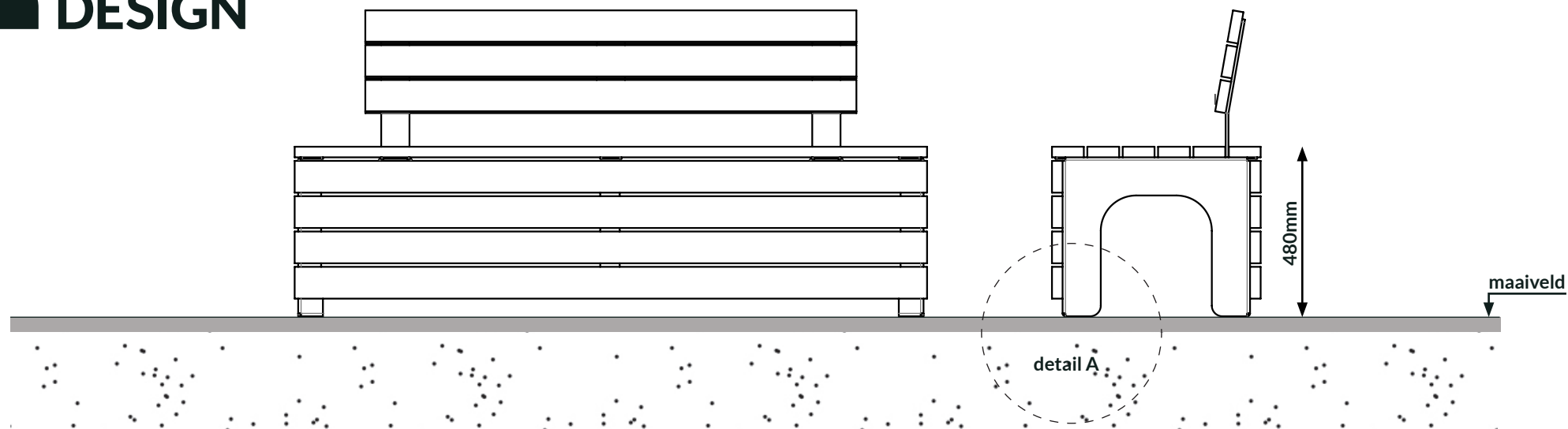
detail A | onder maaiveld
